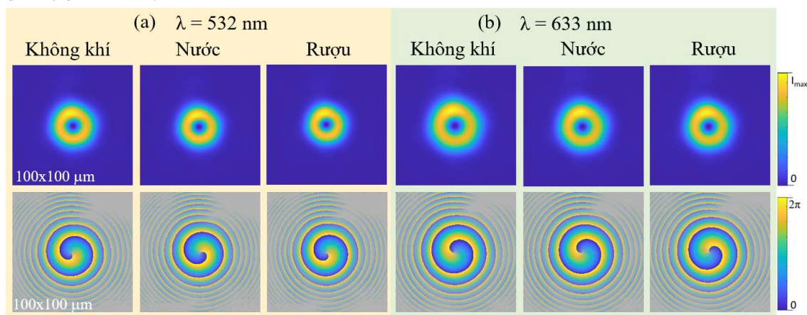
Hình 4. Mô phỏng các xoáy quang hình thành từ cùng một thiết kế vi linh kiện pha xoáy cấu trúc nano trong các môi trường không khí, nước và rượu. Mô phỏng cho bước sóng 532 nm với thiết kế vi linh kiện có độ dày d_{532\text{nm}} = 6.0 \mu\text{m} (a). Mô phỏng cho bước sóng 633 nm với thiết kế vi linh kiện có độ dày d_{633\text{nm}} = 7.7 \mu\text{m} (b)
