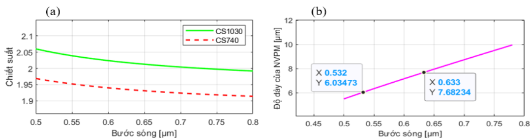
Hình 2. (a) Chiết suất của vật liệu CS740 và CS1030. (b) Độ dày của vi linh kiện được tính toán để tạo xoáy quang bậc cơ bản tại vùng khả kiến
