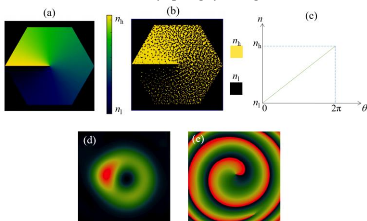
Hình 1. Thiết kế cấu trúc trung tâm của vi linh kiện xoay quang học có bề mặt phẳng với sự phân bố chiết suất biến đổi tuyến tính liên tục lý tưởng theo góc phương vị \theta (a, c) và thiết kế cấu trúc nano tương ứng (b). Mô phỏng xoay quang học với các vi linh kiện này sử dụng vật liệu thủy tinh mềm borosilicate (NC) đã công bố trên [14]: Phân bố cường độ (d) và cấu hình pha (e).
