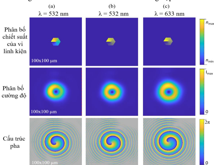
Hình 3. Phân bố chiết suất của các thiết kế vi linh kiện xoáy quang (Hàng trên cùng). Mô phỏng phân bố cường độ ánh sáng (hàng giữa) và cấu hình pha (hàng dưới cùng) trên mặt cắt của xoáy được hình thành khi chiếu sáng vi linh kiện xoáy ở bước sóng \lambda = 532 \text{ nm} (a,b) và 633 \text{ nm} (c)
